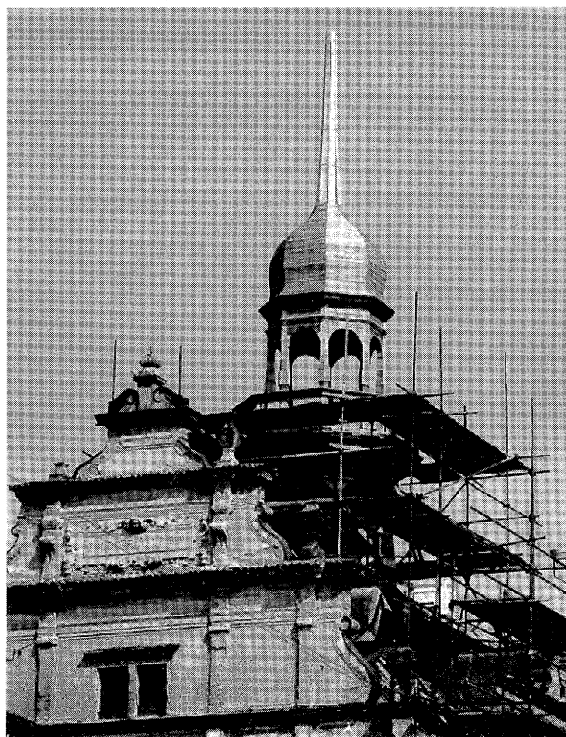
Z opravy bývalého Okresního domu - nový skelet věže po osazení na budovu
