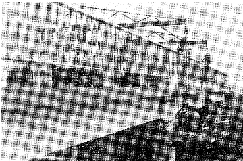
Závěrečné montážní práce na nosnících mostu z předpjatého betonu ve Vřestarech
